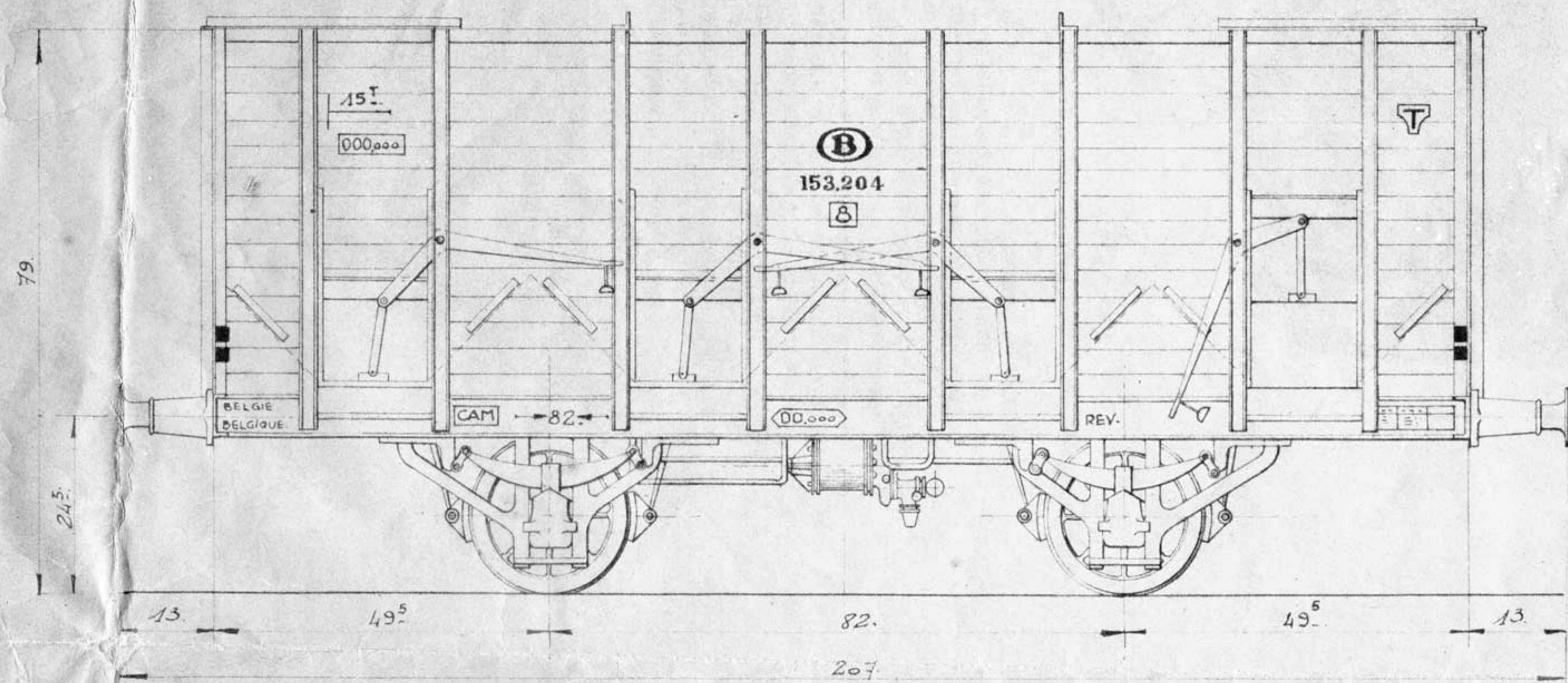
ÉLEVATION
