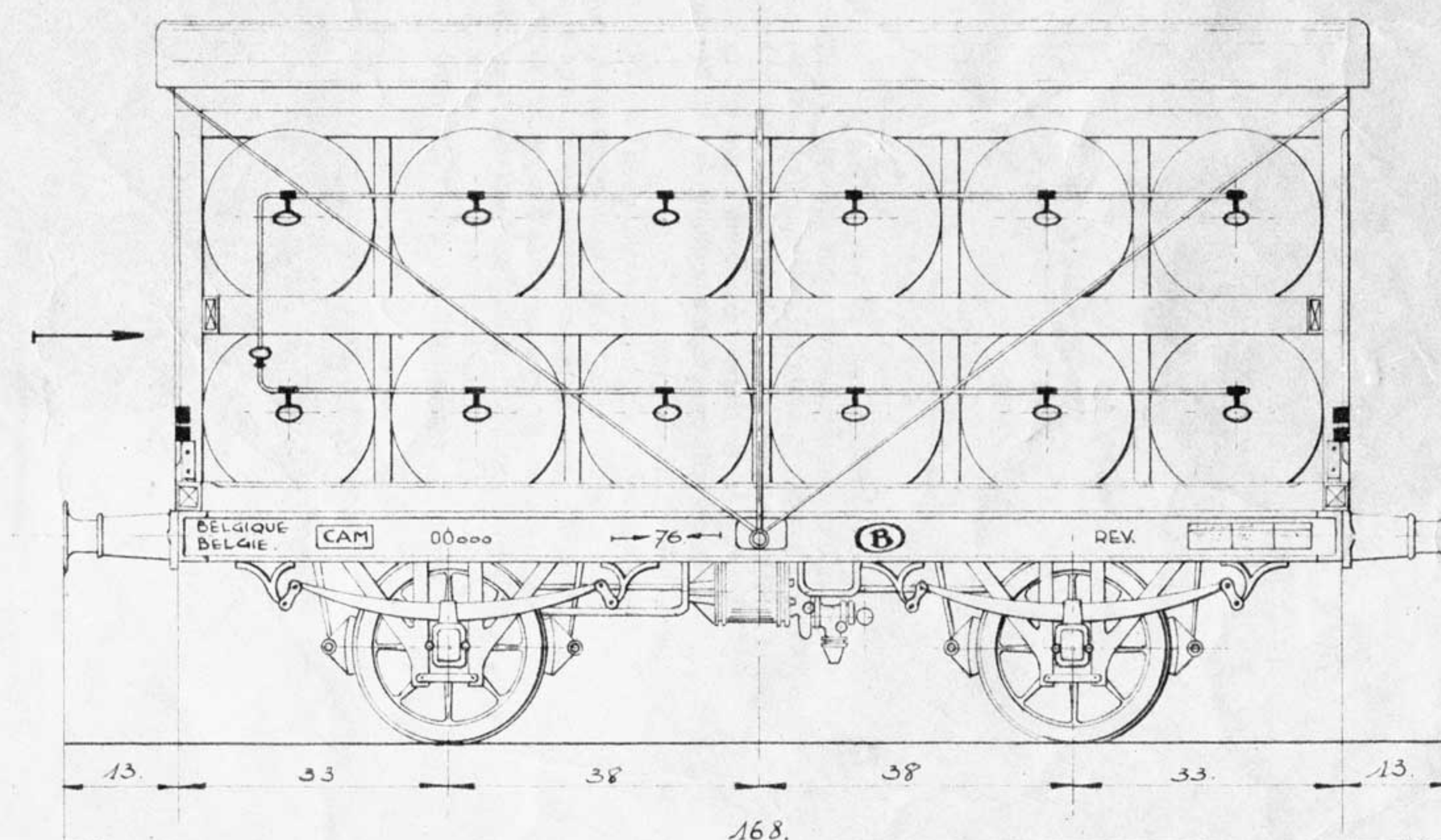
ÉLEVATION
