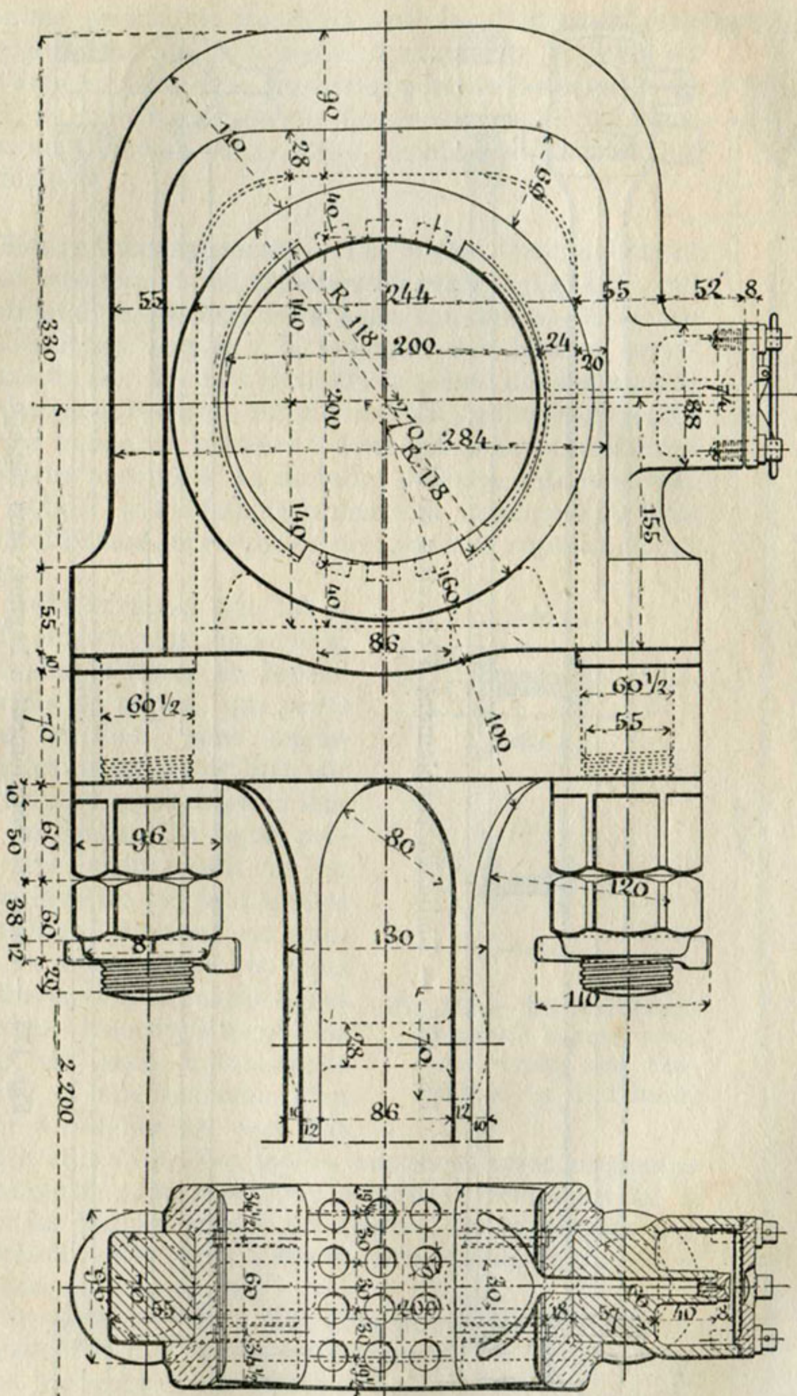
Fig. 131. — Grosse tête de bielle motrice, à chape fileté, des locomotives n o s 963-990 des chemins de fer de l'Ouest (d'après M. Demoulin).
