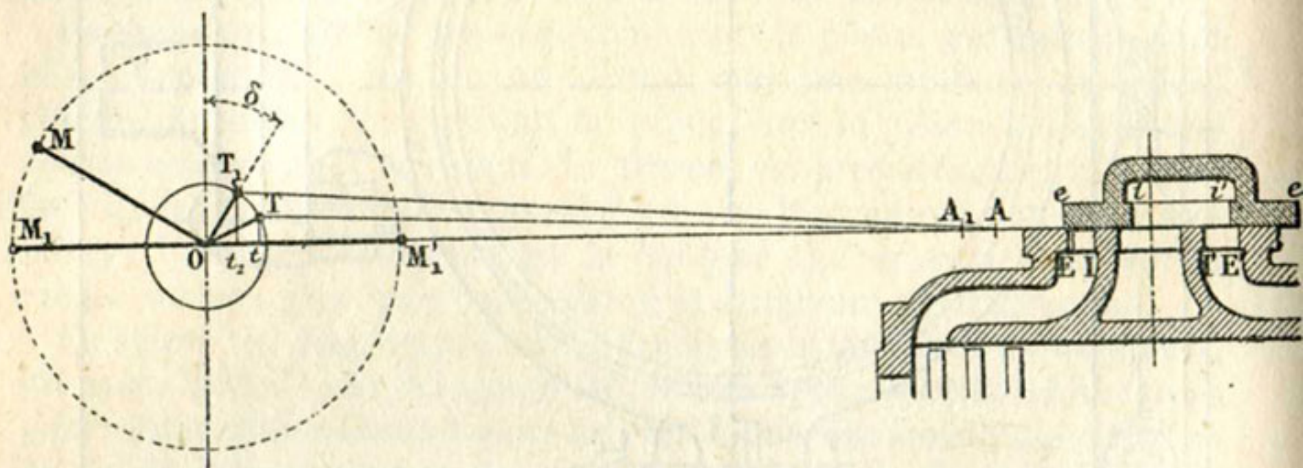
Fig. 149. — Commande du tiroir par un excentrique (la coupe du tiroir et des lumières du cylindre est rabattue sur le plan de la figure par une rotation d'un angle droit).
