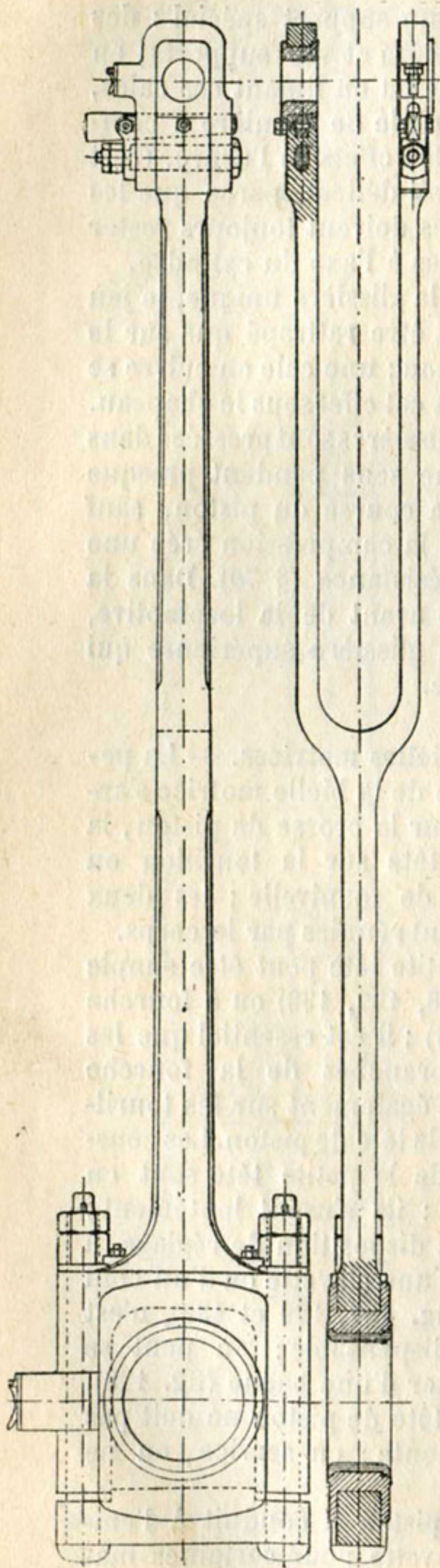
Fig. 127. — Bielle motrice avec petite tête à fourche et à chapes rapportées, et avec grosse tête à cage ouverte et à chapeau.
