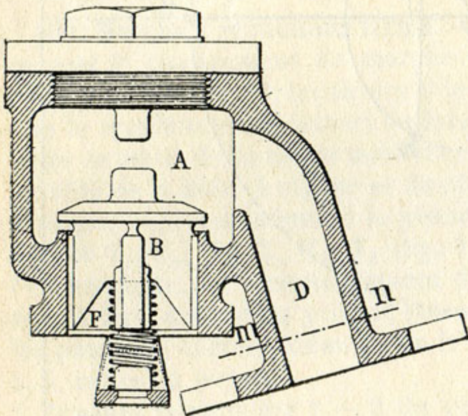
Fig. 188. — Soupape de rentrée d'air montée sur la boîte à vapeur d'un cylindre de locomotive.
