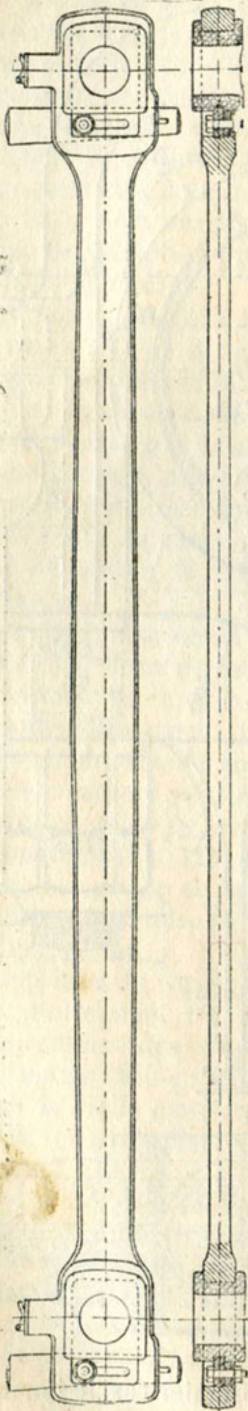
Fig. 132. — Bielle d'accouplement à clavettes de réglage.
