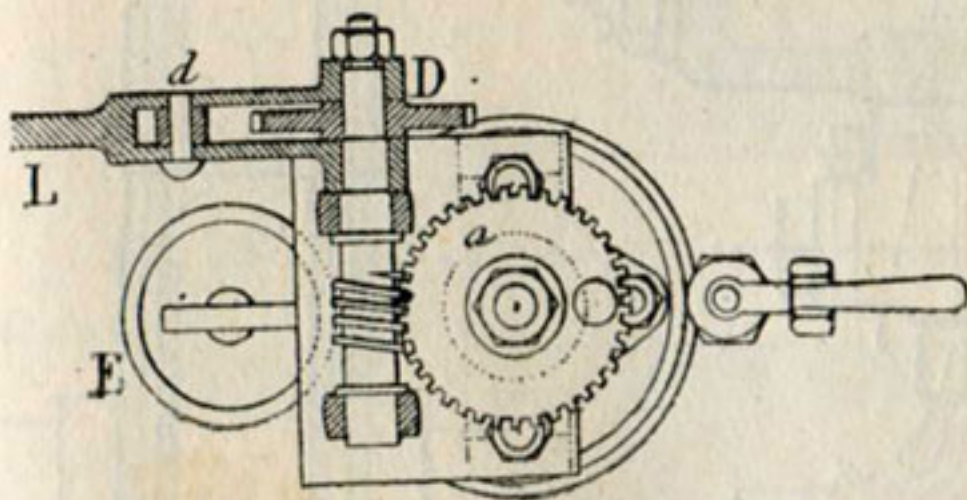
Fig. 115. — Graisseur mécanique Mollerup.
