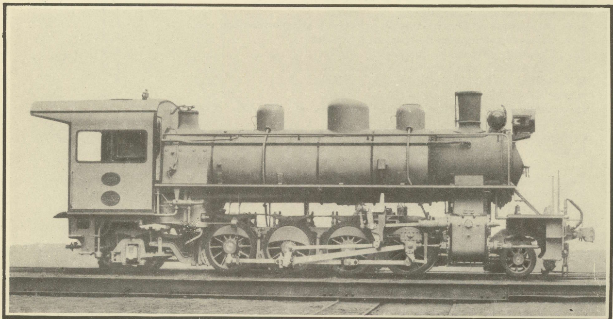
LOCOMOTIVE TYPE MIKADO. — CONSTRUITE PAR LES ATELIERS COCKERILL A SERAING (Belgique), POUR LES CHEMINS DE FER DU B.C.K.
