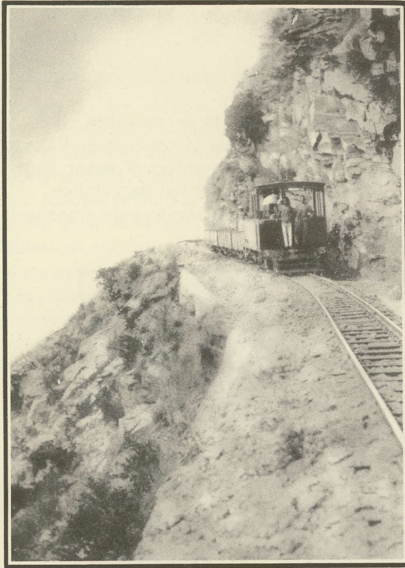
CHEMIN DE FER MATADI-LEOPOLDVILLE LA VOIE AU KILOMÈTRE 2.700
