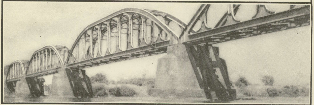
BUKAMA. — PONT RAIL A QUATRE TRAVÉES DU TYPE VIERENDEEL, D'UNE LONGUEUR TOTALE DE 240 MÈTRES, CONSTRUIT SUR LE LUALABA
