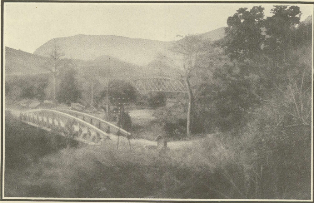
CHEMIN DE FER DE MATADI A LÉOPOLDVILLE — PONTS SUR LA M' POSO. A L'AVANT-PLAN, CELUI DE L'ANCIENNE LIGNE (ÉCARTEMENT 0 m. 765), A L'ARRIÈRE PLAN, CELUI DE LA NOUVELLE LIGNE (ÉCARTEMENT 1 m. 067)
