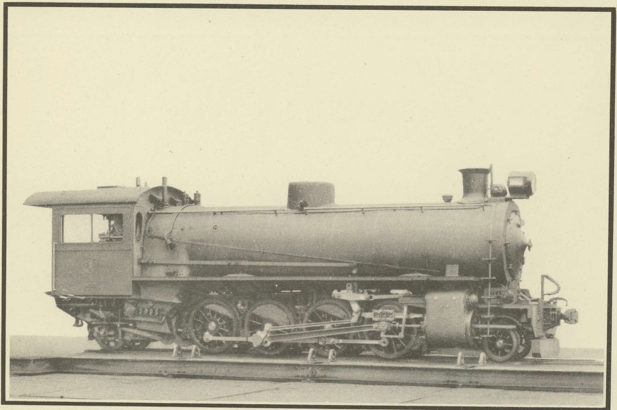
LOCOMOTIVE MIKADO. — CONSTRUITE PAR LA S. A. JOHN COCKERILL A SERAING (Belgique), POUR LE CHEMIN DE FER MATADI-LÉOPOLDVILLE
