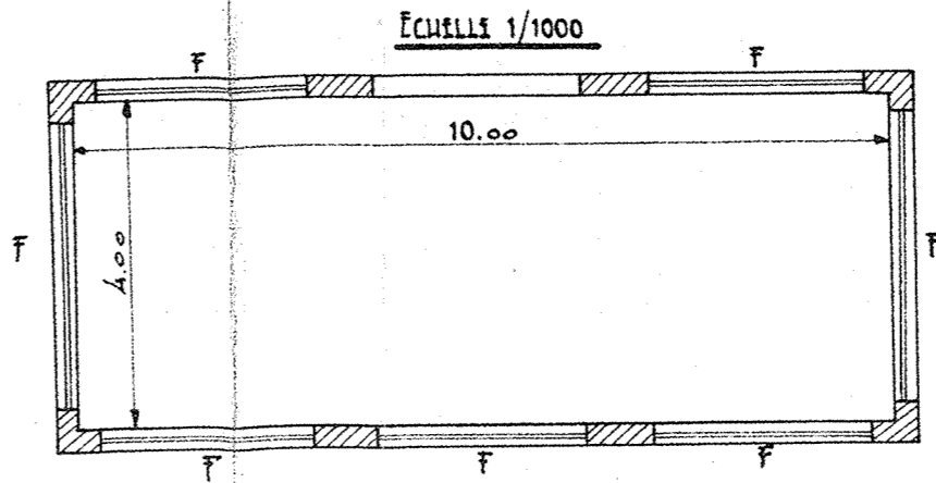
VUE EN PLAN DE L'ABRI À VOYAGEURS Echelle 1/1000.
